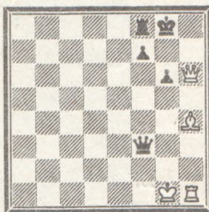
351. Ход белых
