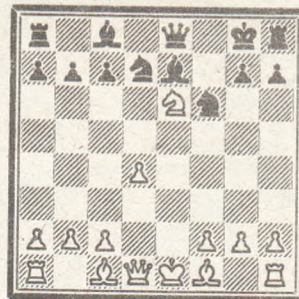
358. Ход белых
