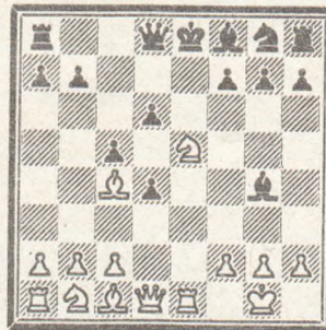
360. Ход черных
