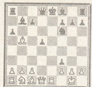
359. Ход черных
