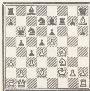
354. Ход белых
