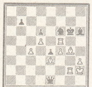
362. Ход белых
